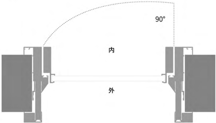
Frame Diagram 框型简图
