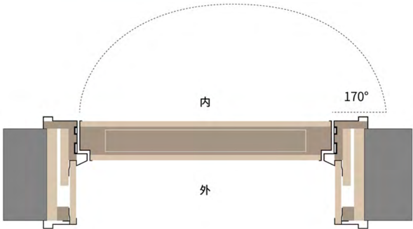
框型简图 Frame Diagram
