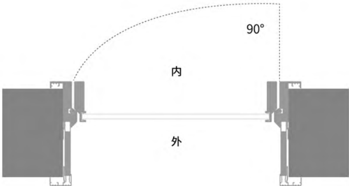
Frame Diagram 框型简图
